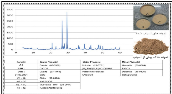
شکل ۵: نتایج حاصل از آزمایش XRD بر روی خاک قلع مورچه خورت (آزمایشگاه شهرک فناوری دانشگاه صنعتی اصفهان، ۱۴۰۳)
