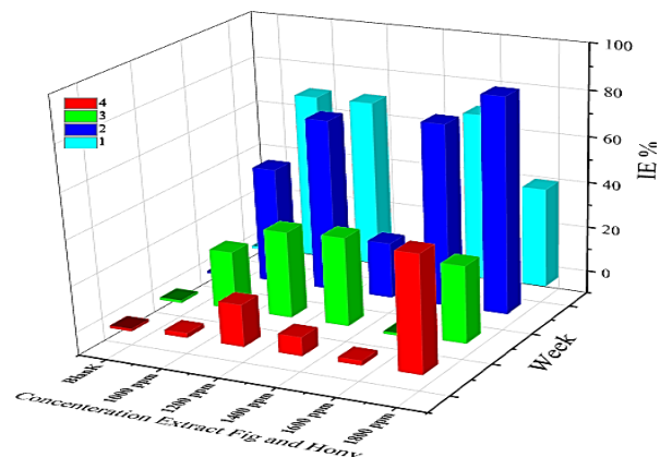
شکل ۴. میزان بازده بازدارندگی عسل کنار با غلظت 1800 ppm و شیره انجیر سفید غلظت با غلظت‌های 1000 تا 1800 ppm بعد از یک تا چهار هفته که با رنگ‌های مشخص در راهنمای منحنی آورده شده است.
