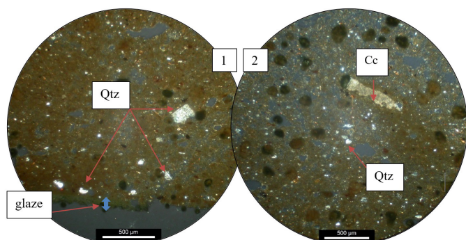
شکل ۵. فتومیکروگراف، نمونه ۱، نور XPL، طول میدان دید 2.7mm، بافت سیلته و ریز دانه، خمیره سفال همگن و قطعات کانی کوارتز به طور پراکنده و محدود در خمیره دیده می شود. فتومیکروگراف، نمونه ۲، نور XPL، طول میدان دید 2.7mm، بافت سیلته، کانی کلسیت همراه با کوارتز در خمیره سفال.
