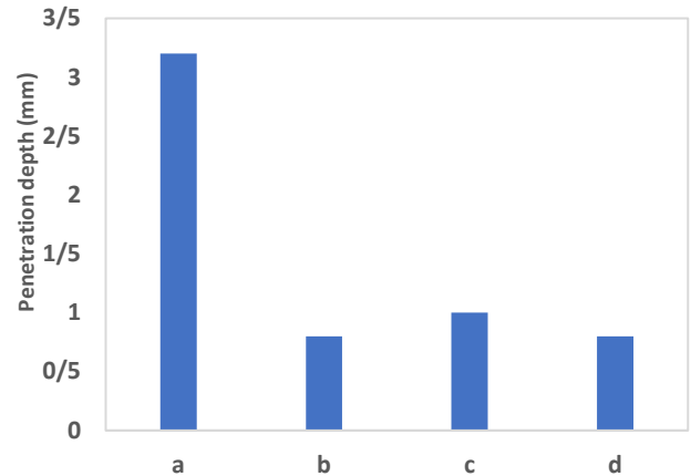
شکل ۳. میزان عمق نفوذ تیمار پلی وینیل بوتیرال بر حسب میلی متر: عمق نفوذ با تیمار پلی وینیل بوتیرال ۱ درصد (a)، میزان عمق نفوذ با تیمار مخلوط 1/5 ، 1/5 درصد پلی وینیل بوتیرال و پارالوید B-72 (b)، میزان عمق نفوذ با تیمار پلی وینیل بوتیرال ۳ درصد (c)، میزان عمق نفوذ با تیمار پلی وینیل بوتیرال ۵ درصد (d).
