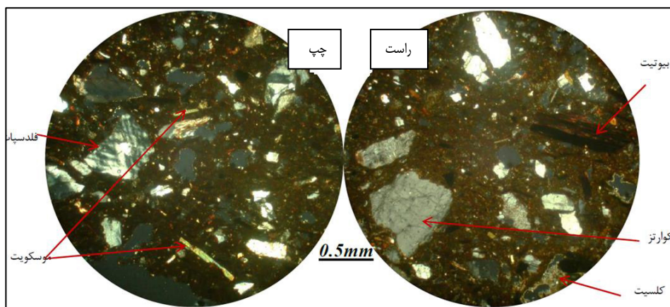
شکل ۱۰. (راست): تصویر میکروسکوپی نمونه ۱۶، نور XPL، طول میدان دید 2.7 mm، بافت پورفیری، کانی‌های کوارتز، فلدسپات و مسکویت به صورت درشت‌بلور، بیوتیت سوخته شده، میکا همراه با کلسیت در خمیره سفال دیده می‌شود. (چپ): تصویر میکروسکوپی نمونه ۱۷، نور XPL، طول میدان دید 2.7 mm، بافت پورفیری، کانی کوارتز
