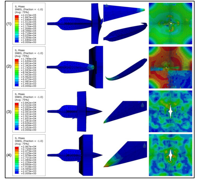
شکل ۹. نمودار تنش مدل L در برخورد: ۱. حالت A.B-S.A، ۲. حالت B.B-S.A، ۳. حالت A.B-L.A، ۴. حالت B.B-L.A Figure 9. The stress charts of model L at the impact in (1) A.B-S.A state, (2) B.B-S.A state, (3) A.B-L.A state, (4) B.B-L.A state.
