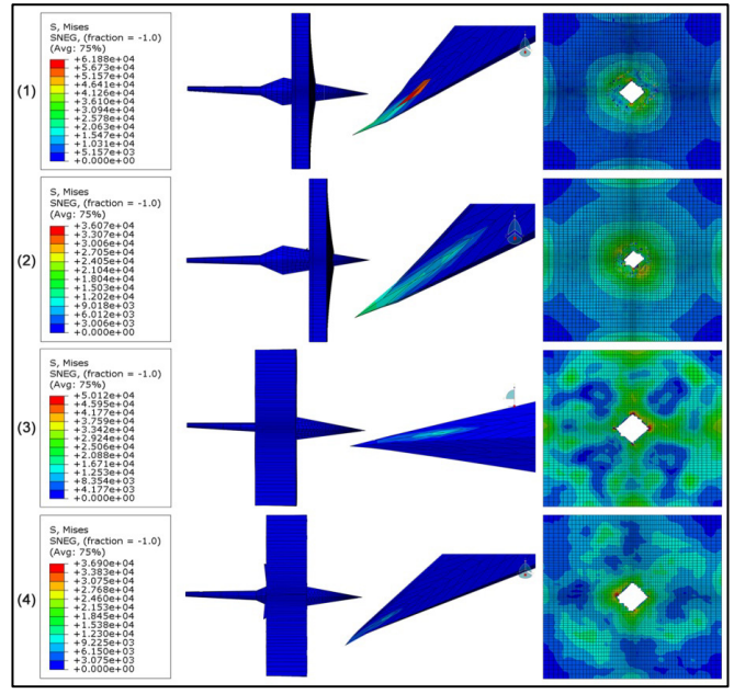
شکل ۸. نمودار تنش مدل B در برخورد: ۱. حالت A.B-S.A، ۲. حالت B.B-S.A، ۳. حالت A.B-L.A، ۴. حالت B.B-L.A Figure 8. The stress charts of Model B at the impact in: (1) A.B-S.A state, (2) B.B-S.A state, (3) A.B-L.A state, (4) B.B-L.A state.
