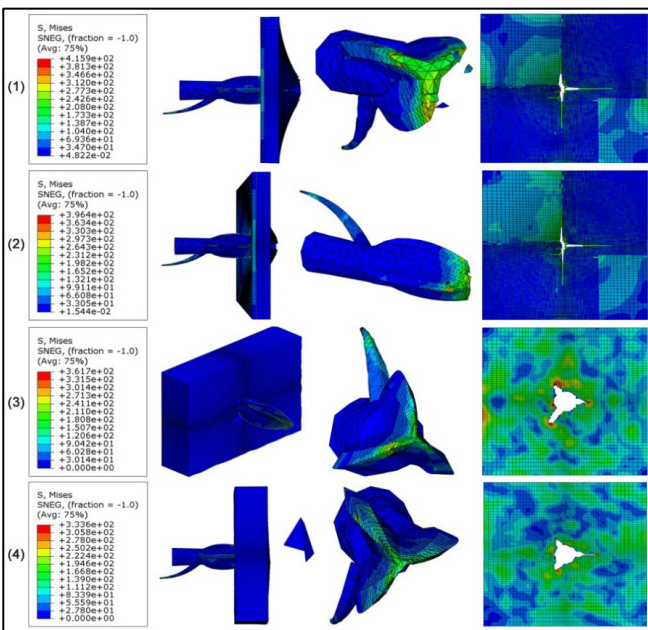
شکل ۱۰. نمودار تنش مدل T در برخورد: ۱. حالت A.B-S.A، ۲. حالت B.B-S.A، ۳. حالت A.B-L.A، ۴. حالت B.B-L.A Figure 10. The stress charts of model T at the impact in (1) A.B-S.A state, (2) B.B-S.A state, (3) A.B-L.A state, (4) B.B-L.A state
