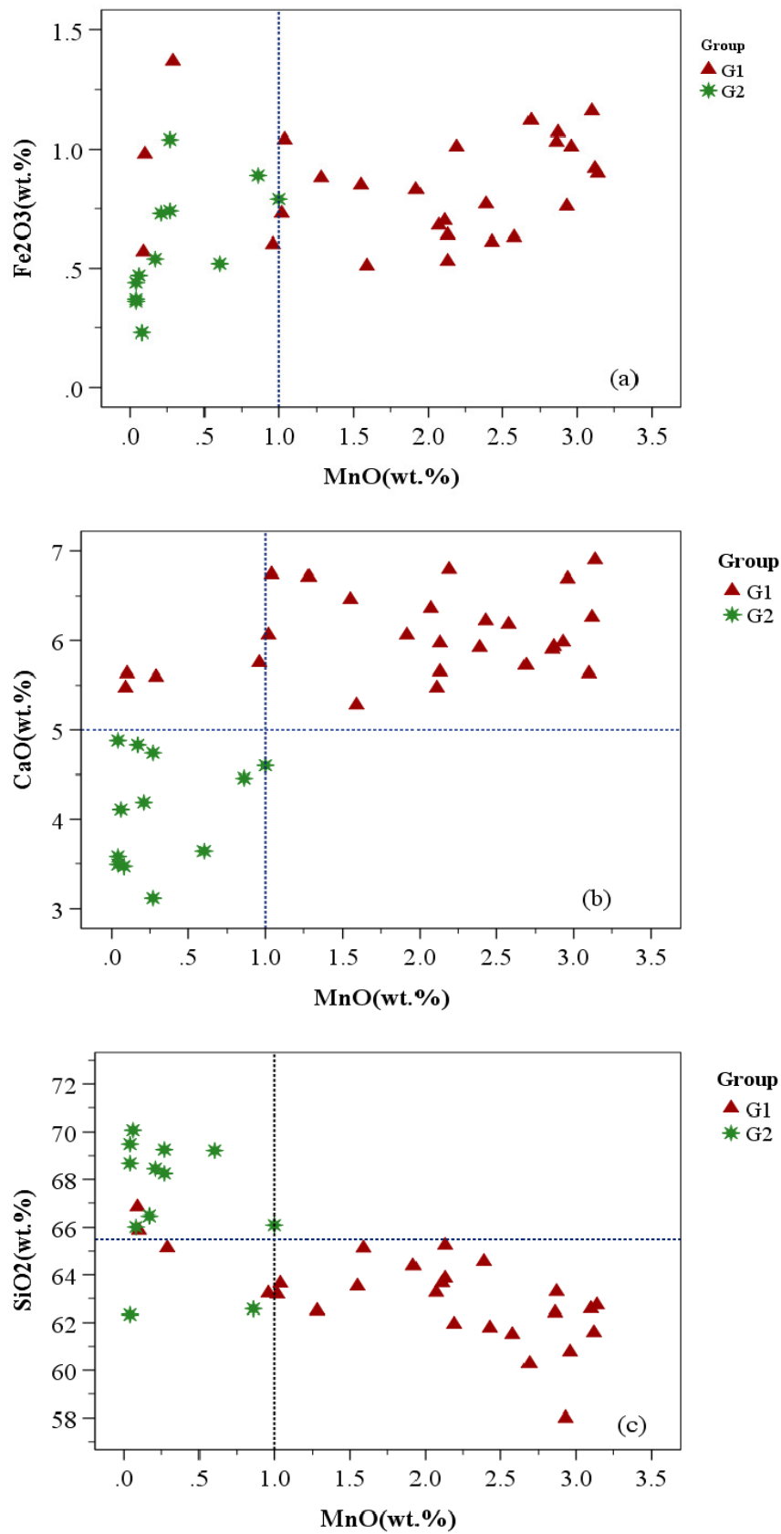
تغییرات اکسید منگنز برحسب اکسید آهن (a) شکل ۷: سیلیسیم در نمونه‌های آنالیز شده از سیمره
