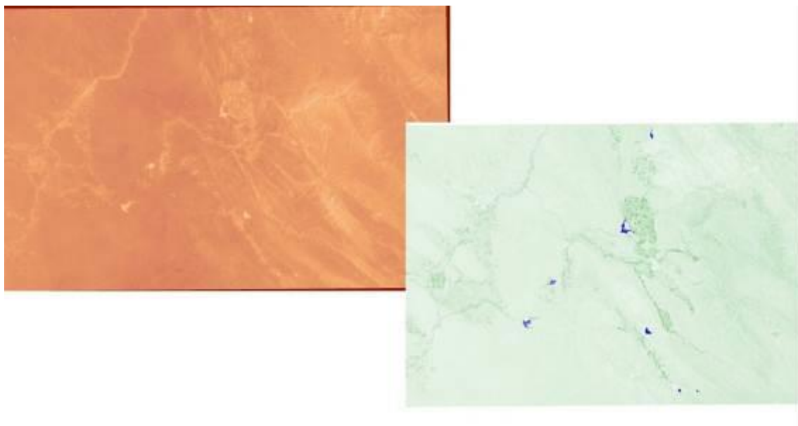
شکل ۵: راست، شاخص NDWI و چپ، شاخص Thermal در کرمانشاه و کلار (ماهواره لندست)
