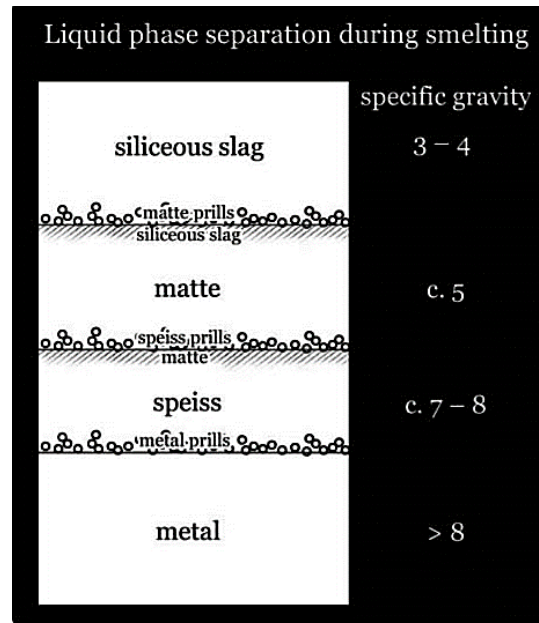
شکل ۳: طرح ساده Keesmann (۱۹۹۱) با توجه به وزن مخصوص ترکیبات، تفکیک جزئی شامل: (۱) سرباره سلیکاتی (۲) مات غنی از مس (یعنی سولفید آهن) مس (۳) اشپایس (۴) مس Fig. 3: Simple design by keesmann. According to the specific gravity of the compounds, the partial separation includes: 1-Silicate slag 2-Matte, i.e sulfide (Iron) of copper 3- Speiss 4- Copper metal
