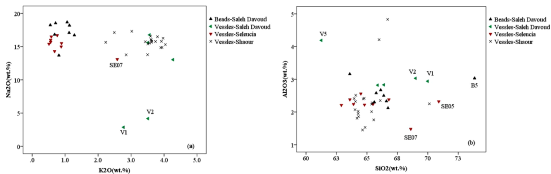
شکل ۶: a- تغییرات درصد وزنی اکسید پتاسیم برحسب اکسید سدیم، b- تغییرات مقدار اکسید سیلیسیم برحسب اکسید آلومینیم در نمونه‌های آنالیز شده از محوطه صالح داود و مقایسه آن‌ها با نمونه‌های شائور در شوش [15] و سلوکیه در عراق [13] Fig. 6: Scatter plot of wt% of (a): K 2 O versus Na 2 O, (b): SiO 2 versus Al 2 O 3 in analyzed sample from Saleh Davoud and their comparison with Shaour glasses in Susa [15] and Selucia in Iraq [13]
