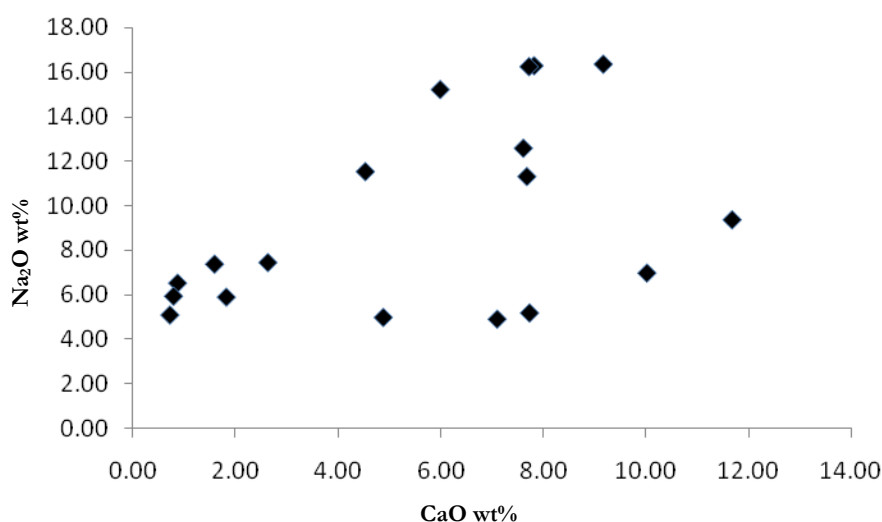
شکل ۳: میزان درصد اکسید سدیم در مقابل اکسید کلسیم در شیشه‌های سدیم-کلسیم-سیلیکات
