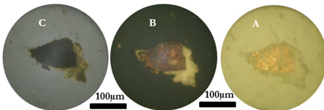
شکل ۱۴: تصاویر میکروسکوپی رنگ طلایی در نور A: پلاریزه، B: عبوری، C: انعکاسی، که وجود کالکوپیریت را نشان می‌دهد. Fig. 14: golden Microscopic Images in the Light: A: Polarizing, B: Reflection C: Transmission, showing the presence of chalcopyrite.
