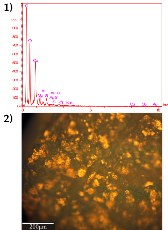
شکل ۹. آنالیز SEM-EDS و عناصر به دست آمده از ذرات طلایی (۱) و تصویر میکروسکوپی انعکاسی از سطح رنگ (۲).
