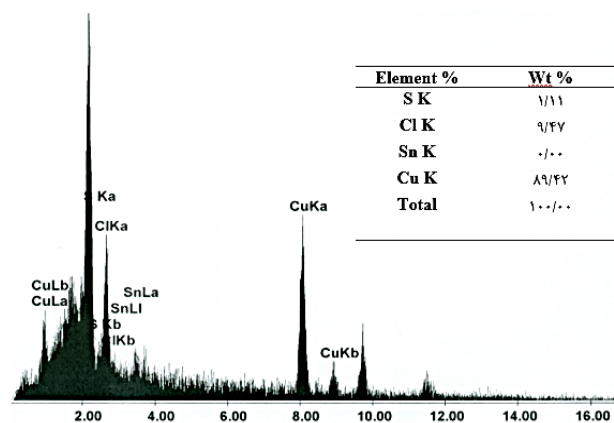
شکل ۶. آنالیز EDX از کوپن شاهد در محلول سدیم کلرید ۰/۵ مولار
