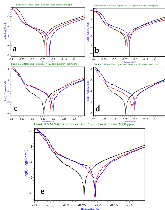
شکل ۲. منحنی پلاریزاسیون تافل با خطوط مشکی مربوط به محیط خورنده سدیم کلرید ۰/۵ مولار. با خطوط قرمز نشان‌دهنده شیریه انجیر سفید، آبی منحنی هم‌افزا عسل کنار و شیریه انجیر سفید (الف) منحنی پلاریزاسیون تافل مربوط به عسل کنار با غلظت ۱۸۰۰ ppm و انجیر سفید با غلظت ۱۰۰۰ ppm (ب) منحنی پلاریزاسیون تافل مربوط به عسل کنار با غلظت ۱۸۰۰ ppm و شیریه انجیر سفید با غلظت ۱۲۰۰ ppm (ج) منحنی پلاریزاسیون تافل مربوط به عسل کنار با غلظت ۱۸۰۰ ppm و شیریه انجیر سفید با غلظت ۱۴۰۰ ppm (د) منحنی پلاریزاسیون تافل مربوط به عسل کنار با غلظت ۱۸۰۰ ppm و شیریه انجیر سفید با غلظت ۱۶۰۰ ppm (ه) منحنی پلاریزاسیون تافل مربوط به عسل کنار با غلظت ۱۸۰۰ ppm و شیریه انجیر سفید با غلظت ۱۸۰۰ ppm
