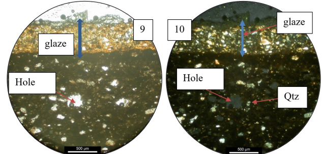
شکل ۹. فتومیکروگراف، نمونه ۹، نور PPL، طول میدان دید ۲.۷mm، بافت ناهمگن، لایه لعاب در بالای تصویر که دو لایه لعاب شیشه ای همراه با لایه متشکل از کوارتز و مذاب سیلیسی که بر روی بدنه قرار دارد. در این نور فضای خالی به رنگ روشن است. فتومیکروگراف، نمونه ۱۰، نور XPL، طول میدان دید ۲.۷mm، بافت ناهمگن. همان تصویر ۹ در نور متقاطع است.
