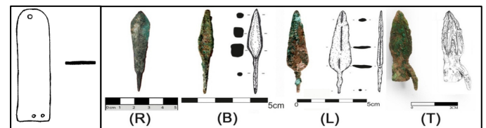
شکل ۲. نمونه‌های مورد آزمایش: B. زبانه دار با تیغه‌ی هرمی شکل (بادکین) (Dehpahlavan, 1395). L. زبانه‌دار دوطبقه با تیغه‌ی برگ‌ی شکل (ibid) T. سه پره‌ی سوکتی با خار روی سوکت (Dehpahlavan, 1398). R. زبانه‌دار دو لبه با تیغه‌ی لوزی شکل S.A. نمونه پولک برنزی از زره پولکی (Stronach, 1958)
