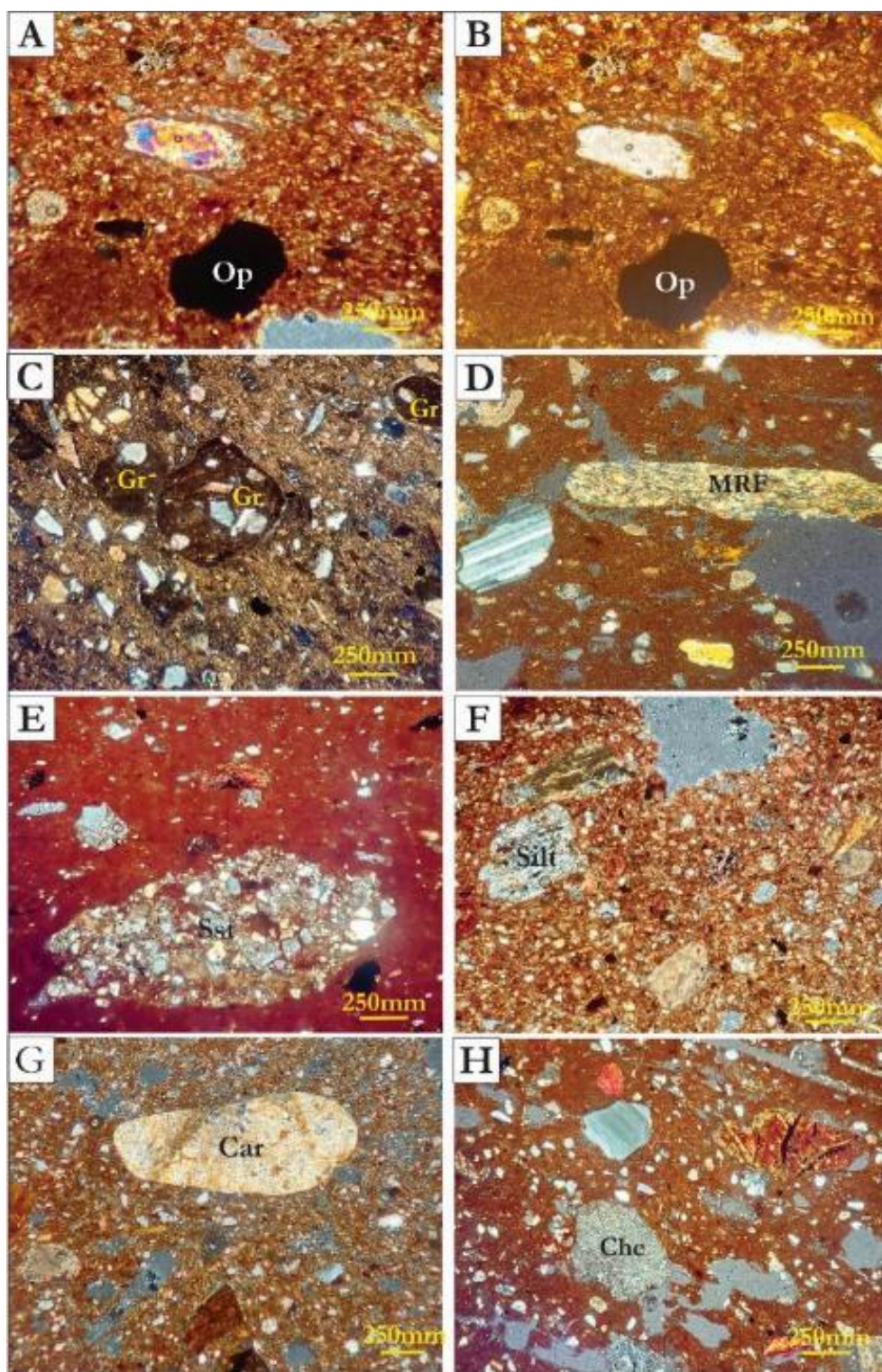
شکل ۵: تصاویر میکروسکوپی از انواع مواد افزودنی شناسایی شده (بزرگنمایی ۱۰×)، A) کانی سنگین تیره (احتمالاً مگنتیت) (Op) نور پلاریزه متقاطع، B) همان تصویر در نور پلاریزه موازی، کانی سنگین اپاک در هر دو نور تیره هستند، C) گراگ یا خرده سفال (Gr)، D) خرده سنگ دگرگونی اسلیتی (MRF)، E) خرده سنگ رسوبی ماسه سنگی (Sst)، F) خرده سنگ رسوبی سیلتستونی (Silt)، G) خرده سنگ رسوبی کربناته (Car) و H) خرده سنگ رسوب چرتی (Che)، تصاویر C تا H در نور پلاریزه متقاطع عکس‌برداری شده است.
