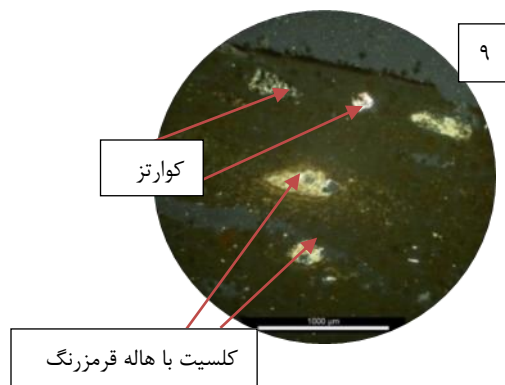
شکل ۱۰: تصویر میکروسکوپی از نمونه 7-1401، نور XPL، طول تصویر 2.7mm، کانی کوارتز همراه با کلسیت در مرکز تصویر. وجود هاله قرمز رنگ در حاشیه کانی کلسیت می‌تواند نشانگر واپاشی این کانی باشد. خمیره سفال کاملاً متفاوت، همگن و ترکیب غیر کربناتی دارد.
