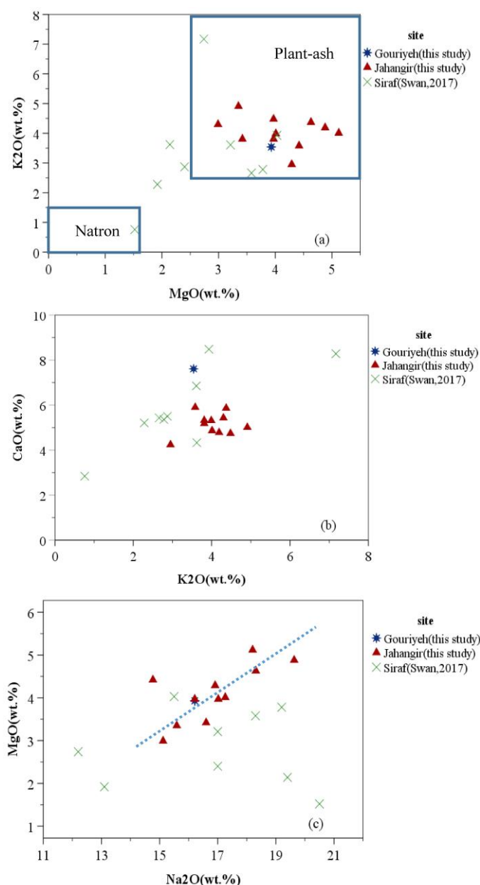
شکل ۳: (a) تغییرات درصد وزنی اکسیدمنیزیم برحسب اکسیدپتاسیم، (b) تغییرات درصد وزنی اکسیدپتاسیم برحسب اکسیدکلسیم، (c) تغییرات درصد وزنی اکسیدسدیم برحسب اکسیدمنیزیم در الگوهای آنالیز شده از گنبد جهانگیر، تپه گوریه و سیراف. همبستگی خطی بین ناخالصی‌های موجود در سودای استفاده شده در نمونه‌های گنبد جهانگیر با خطچین آبی رنگ در شکل نشان داده شده است.
