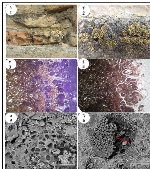
شکل ۵: میکروارگانیسم‌های عامل فرسودگی زیستی: (۱-۲) گل‌سنگ‌های عامل فرسودگی زیستی روی سطح آجری؛ (۳-۴) تصویر میکروسکوپ پلاریزه از نفوذ و مینرالیزاسیون بستر آجری توسط گل‌سنگ‌ها؛ (۵-۶) تصویر میکروسکوپ الکترونی از نفوذ و ایجاد شبکه هیفی با بستر آجری ۲۰ μm توسط گل‌سنگ‌ها با بزرگ‌نمایی
