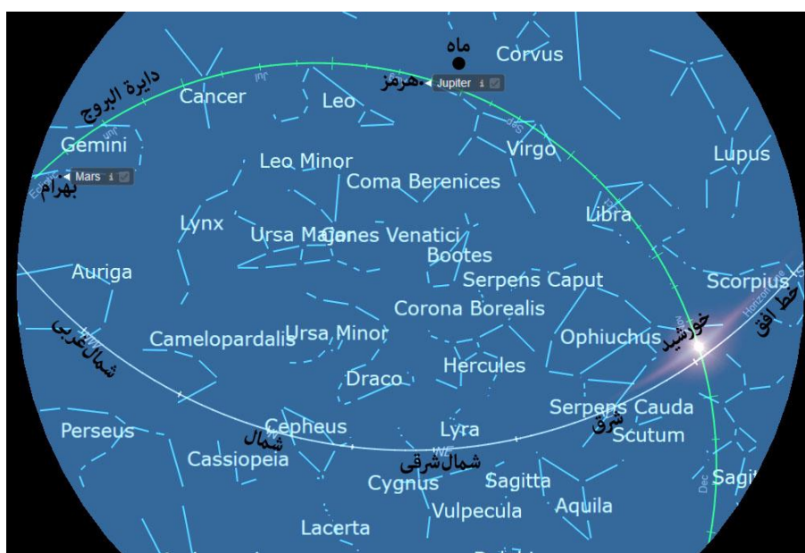
شکل ۲۲: شبیه‌سازی آسمان شهر گور در برنامه استاری‌نایت. صبح‌گاه ۲۲ نوامبر سال ۲۲۴ میلادی، ساعت ۶:۵۰ صبح. موقعیت آفتاب در افق جنوب‌شرقی (که در حال طلوع است)، هرمزد در شمال (مایل به شرق)، و بهرام در غرب (مایل به شمال).
