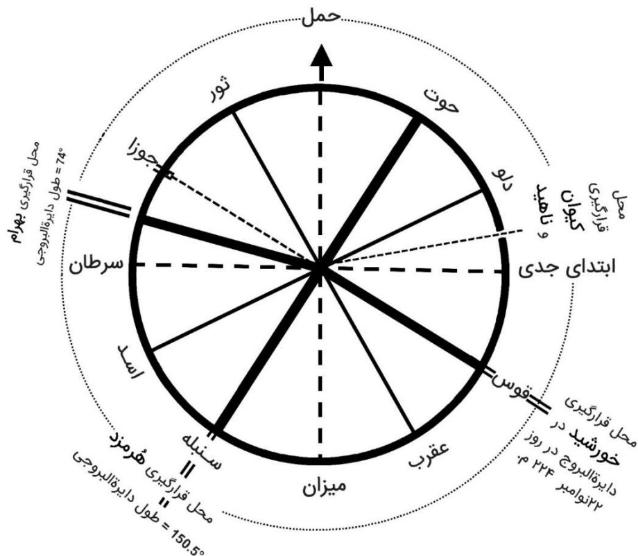
شکل ۲۳: جایگاه خورشید، هرمزد، بهرام، کیوان و ناهید، برحسب طول دایره البروجی هر کدام در روز ۲۲ نوامبر سال ۲۲۴ میلادی. دوازده خانه (بُرج) ۳۰ درجه‌ای، که چون جدی، طالع می‌شود، خورشید ۳۰ درجه پایین‌تر از آن در ابتدای بُرج نیمسب (قوس) است، بهرام در دو پیکر (جوزا)، و هرمزد در ابتدای خوشه (سنبله).
