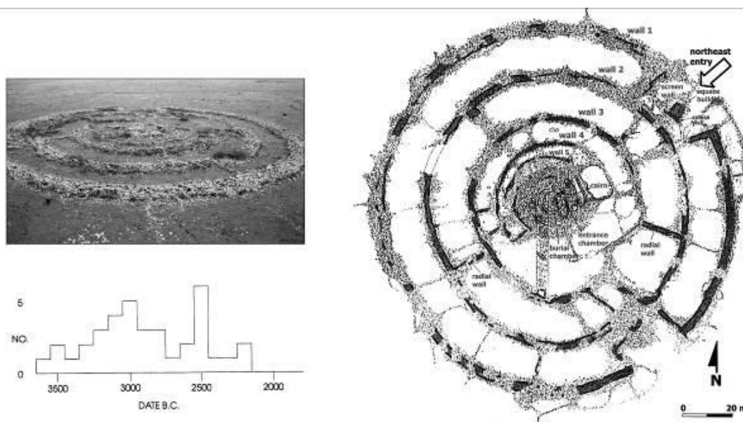
شکل ۱۳: رجم الهیری در بلندی‌های جولان. ورودی شمال شرقی، رو به جایگاه طلوع خورشید در انقلاب تابستانی است. توزیع زمانی هم-ترازی‌های ستاره‌ای (از ۴۰۰۰ تا ۲۰۰۰ قبل از میلاد) که بهترین تناسب را با زاویه‌های سمتی دیواره‌های شعاعی مجموعه دارد، تجمعی را در حدود ۳۰۰۰ قبل از میلاد نشان می‌دهد (Aveni & Mizrachi, 1998).
