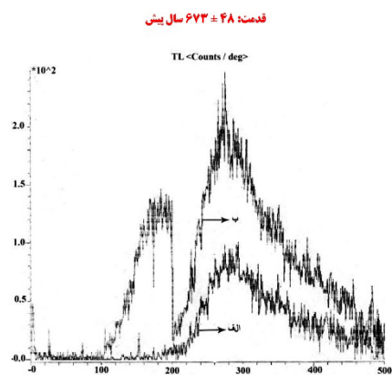
الف- نمودار ترمولومینسانس طبیعی نمونه ب- نمودار ترمولومینسانس نمونه پس از پرتو دهی با چشمه بتا
