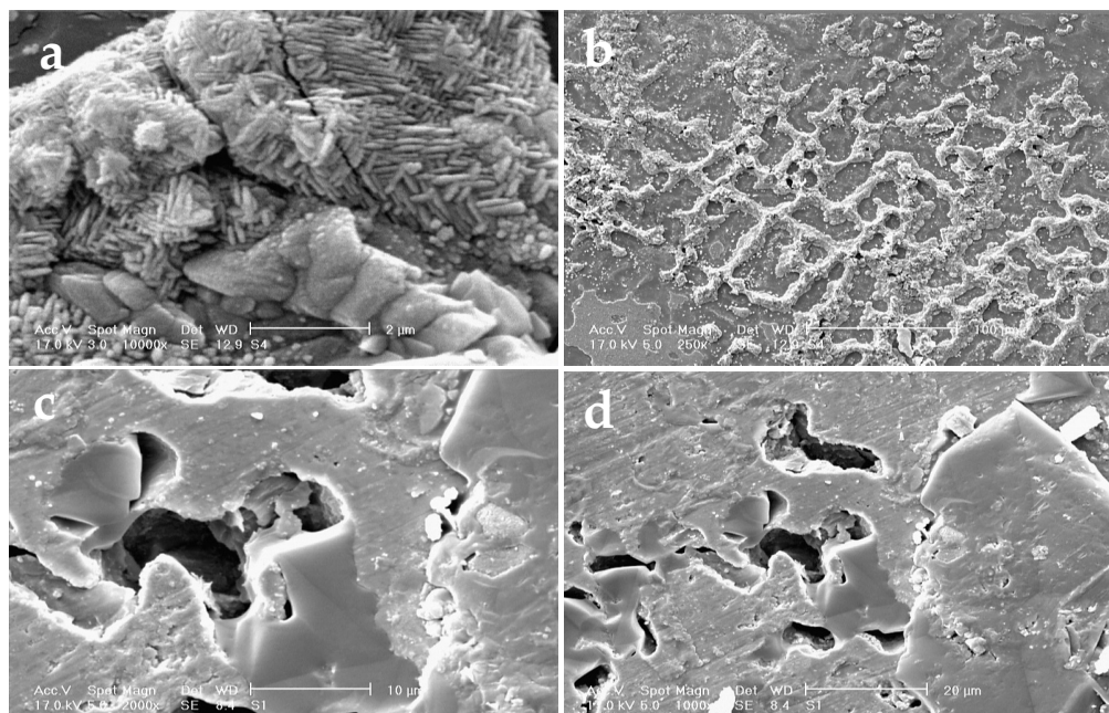
شکل ۵. تصاویر SEM (الف و ب) از کوپن در حضور محلول 0.5\text{ M} سدیم کلرید بعد از یک ماه، تصاویر (ج و د) از کوپن در حضور محلول ترکیبی عسل با غلظت ۱۸۰۰ ppm و شیره انجیر با غلظت ۱۸۰۰ ppm در محلول 0.5\text{ M} سدیم کلرید بعد از یک ماه
