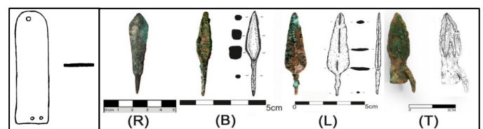
شکل ۲. نمونه‌های مورد آزمایش: B. زبانه دار با تیغه‌ی هرمی شکل (بادکین) (Dehpahlavan, 1395). L. زبانه‌دار دوبله با تیغه‌ی برگی شکل (ibid) T. سه پره‌ی سوکتی با خار روی سوکت (Dehpahlavan, 1398). R. زبانه‌دار دو لبه با تیغه‌ی لوزی شکل S.A. نمونه پولک برنزی از زره پولکی (Stronach, 1958)
