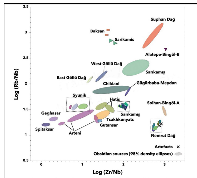
شکل ۵. نمودار مقایسه زیر کونیوم به روییدیوم ( Zr/Nb ) و روییدیوم به نیوبیوم
