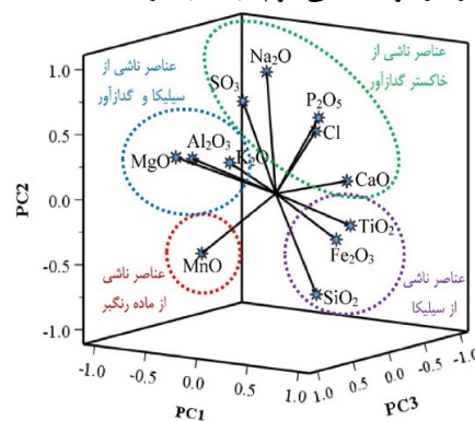
شکل ۷. عناصر و پارامترهای شرکت داده شده در آنالیز فاکتوری و میزان تأثیر این عناصر در پارامترهای پنهان مؤثر در طبقه‌بندی نمونه‌های مورد بررسی.
