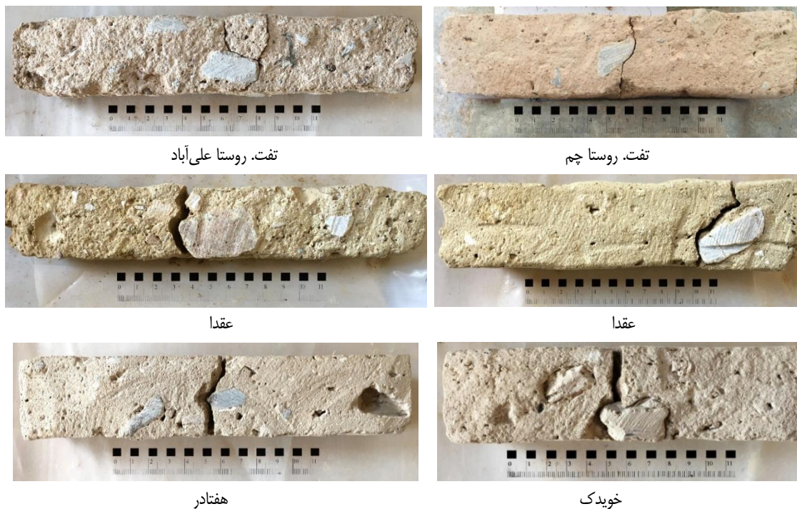
شکل ۳: مسیر شکست در نمونه‌های منشوری تحت آزمون مقاومت خمشی
