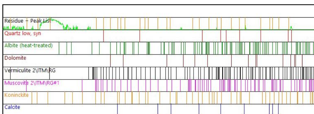
شکل ۱۲: الگوهای فازبازی آزمایش کانی‌شناسی XRD
