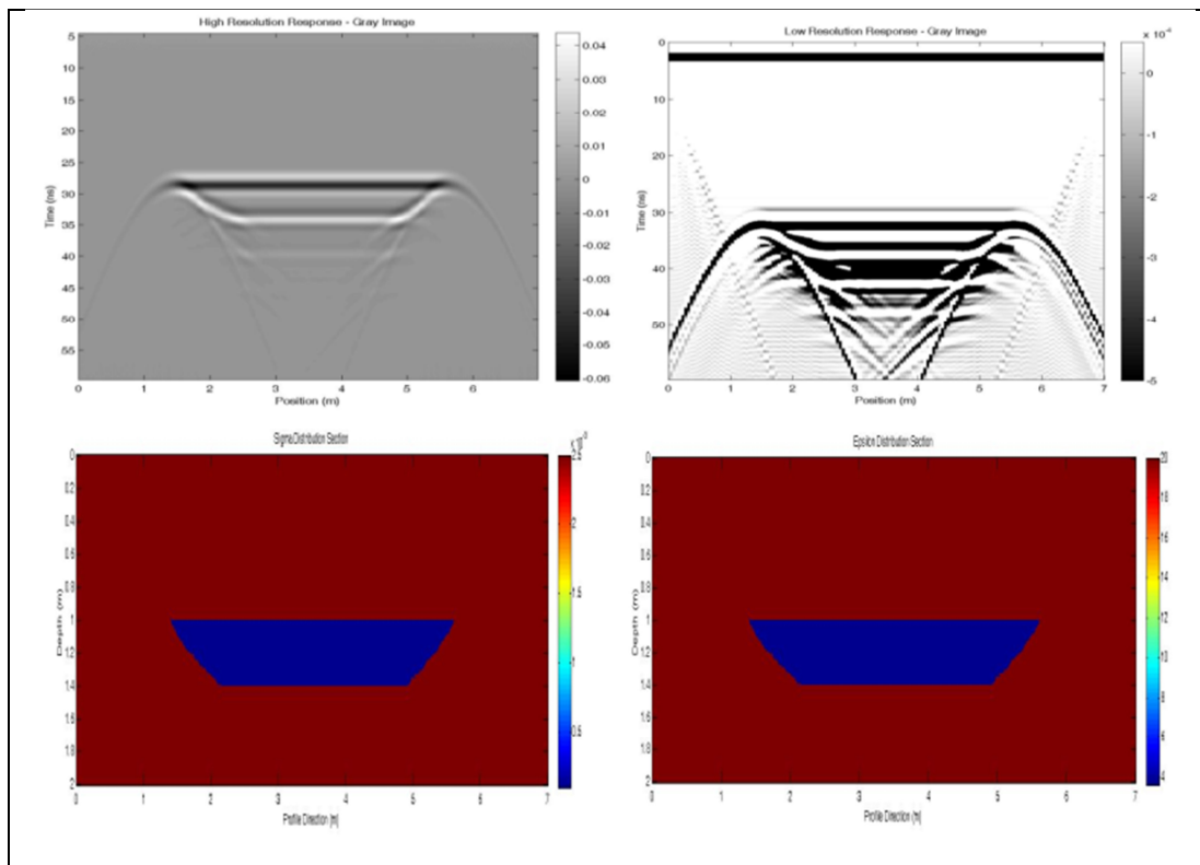
شکل ۸: مدل هندسی و فیزیکی شامل چند ضلعی دوبعدی در قسمت پایین شکل و پاسخ سامانه GPR در قسمت بالای شکل (تفکیک‌پذیری بالا در سمت راست و تفکیک‌پذیری پایین در سمت چپ)
