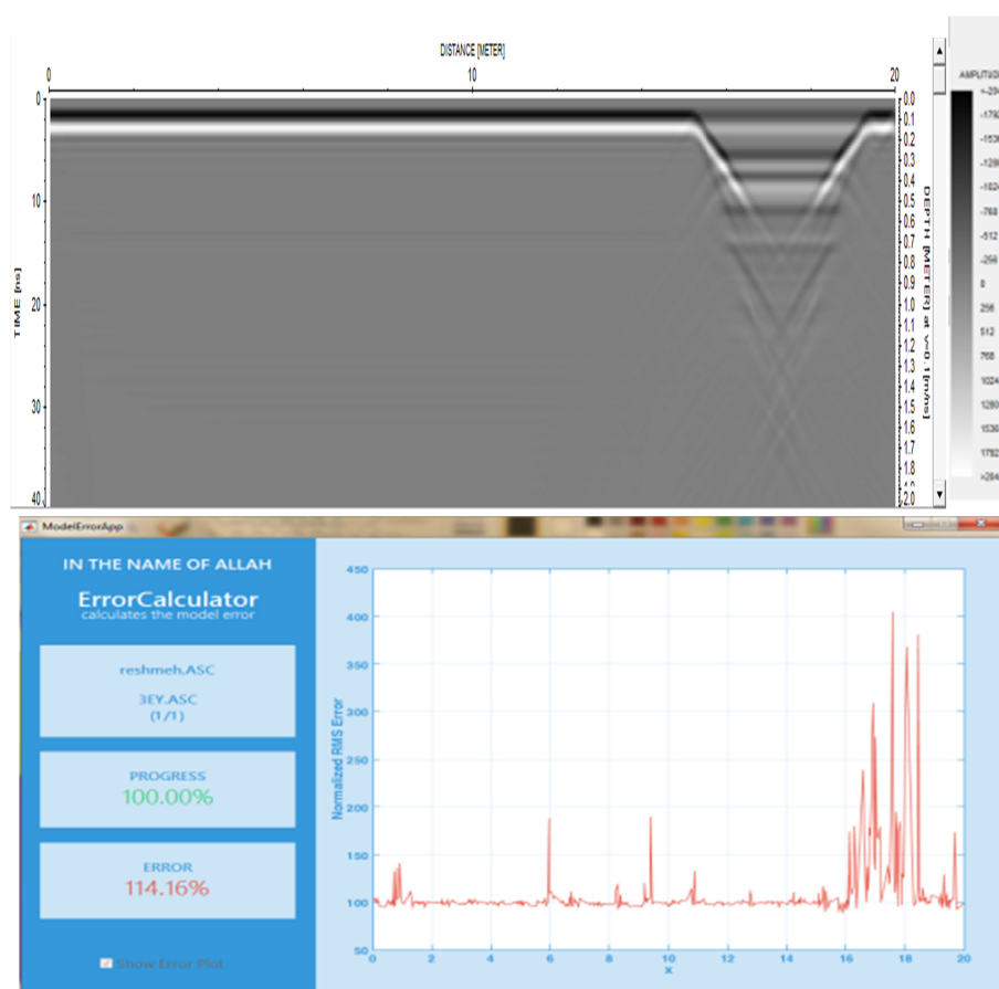
شکل ۹: مدل زمین با بیش‌ترین شباهت به مقطع حاصل از برداشت داده‌های صحرایی در منطقه تپه حصار دامغان همراه با میزان خطای به‌دست آمده
