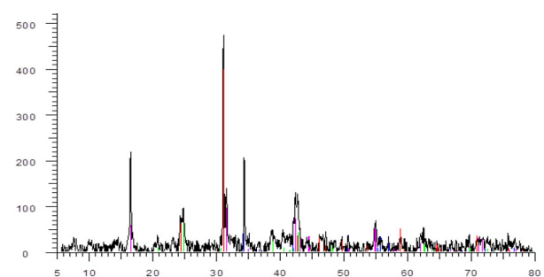
شکل ۲۶. نتایج حاصل از طیف‌سنجی آنالیز XRD Figure 26. Results from XRD analysis spectroscopy
