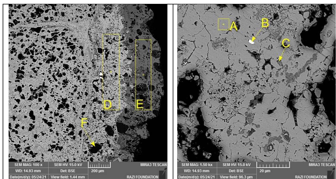
شکل ۱۲: نمونه‌ی SEM-EDS, BM4 با آشکارساز BSE ریزساختار فلز و محصولات و آنالیز نقاط
