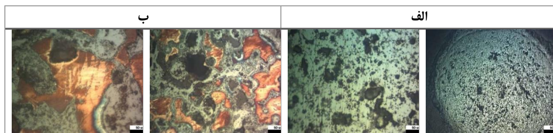
شکل ۵: (الف) نمونه BM1 خلل فرج، محصولات خوردگی، آخال‌های سربی؛ (ب) نمونه BM2 حفره‌ها و خلل فرج، خوردگی مرزدانه‌ای، نواحی به رنگ نارنجی حاوی اکسیدهای مس
