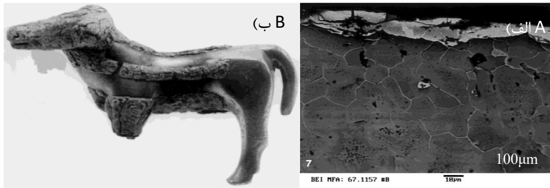
شکل ۹: الف) تصویر SEM از گاو هورز تپه که وجود فاز \gamma به صورت گسترده در سطح نشان‌دهنده پوشش سماتاسیون در سطح این اثر است. ب) گاو به دست آمده از هورز تپه.
