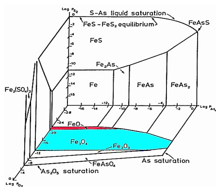
شکل ۴: موقعیت حوزه‌های پایداری فازهای مختلف در سیستم Fe-As-O-S در ۹۷۳ درجه کلوین در فشارهای جزئی مختلف اکسیژن، گوگرد و آرسنیک. اقتباس شده از چاکرابورتی و لینچ [82].
