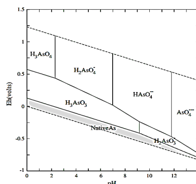
شکل ۱: دیاگرام Eh-pH برای سیستم As-O-H در 25^\circ\text{C} و فشار ۱ bar. \Sigma\text{As} در 106- تنظیم شده است.
