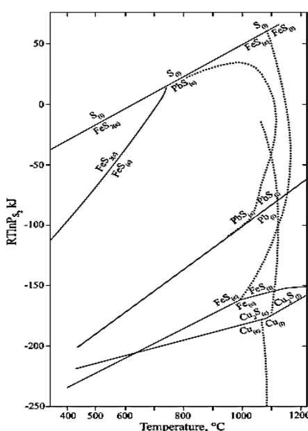
شکل ۵: سبک الینگهام برای آهن، مس و سرب در ارتباط با گوگرد. باز ترسیم شده [86] نشان می‌دهد که در دماهای بالاتر از حدود 650^\circ\text{C} ، خط واکنش \text{Cu}_2\text{S} - \text{Cu} در فشارهای جزئی کمتر است گوگرد از خط \text{FeS} - \text{Fe} ، نشان می‌دهد که مس در مقایسه با آهن ترجیحاً با گوگرد واکنش می‌دهد.
