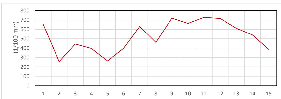
شکل ۳: میانگین منحنی پهنای دواير رشد ستون‌های مسجد قرمز بناب
