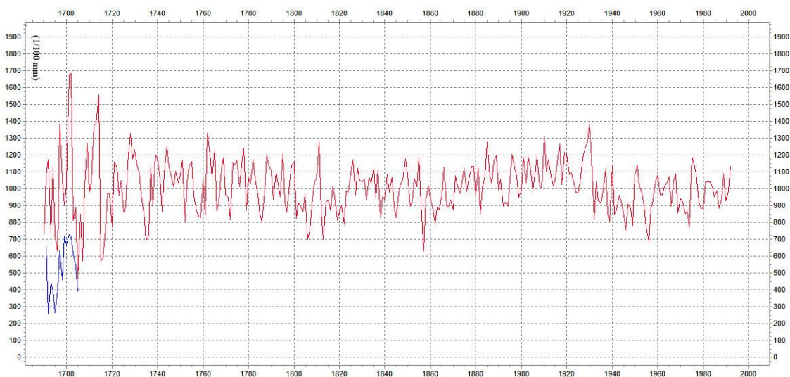
شکل ۹: منحنی میانگین رشد ستون‌های مسجد قرمز در کنار منحنی رویش شرق آناولی (Kuniholm, 2002)
