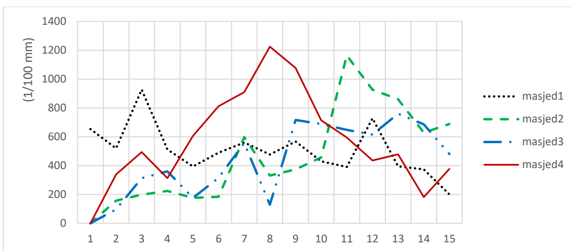
شکل ۲: منحنی رشد نمونه چوب ستون‌های مسجد قرمز بناب
