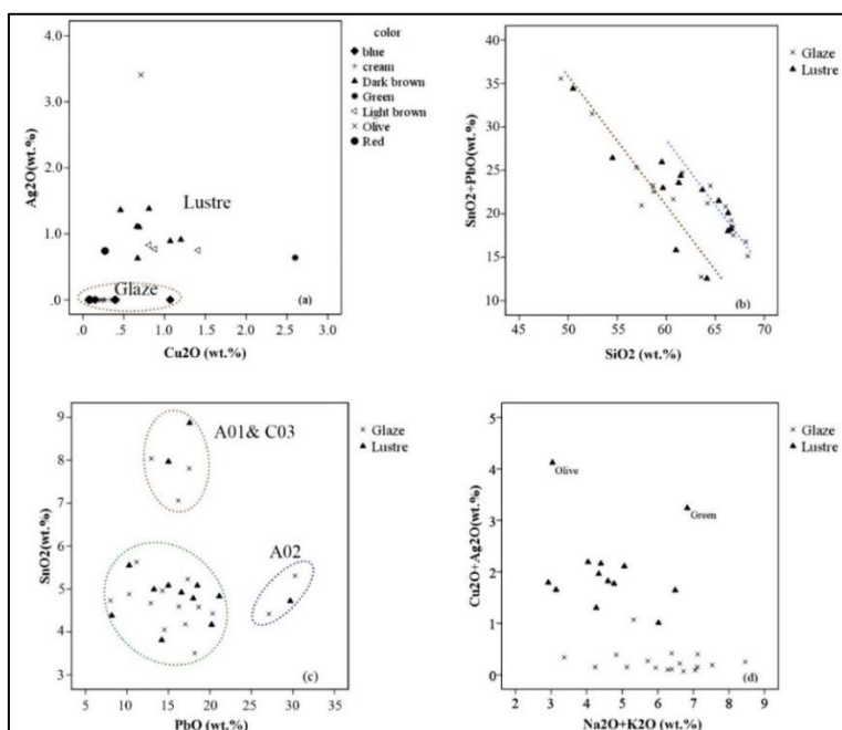
شکل ۱۰: a- تغییرات درصد وزنی اکسید مس برحسب اکسید نقره برای رنگ‌های مختلف زرین‌فام و همچنین لعاب‌های زمینه، b- تغییرات درصد وزنی اکسید مس برحسب اکسید سلیسیم برحسب مجموع اکسیدهای سرب و قلع برای لعاب‌های زرین‌فام و زمینه، c- تغییرات درصد وزنی اکسید سرب برحسب اکسید قلع برای لعاب‌های زرین‌فام و زمینه، d- تغییرات درصد وزنی مجموع اکسیدهای سدیم و پتاسیم برحسب درصد وزنی مجموع اکسیدهای مس و نقره جهت بررسی فرایند تبادل یونی در فرایند ساخت لایه‌های زرین‌فام.
