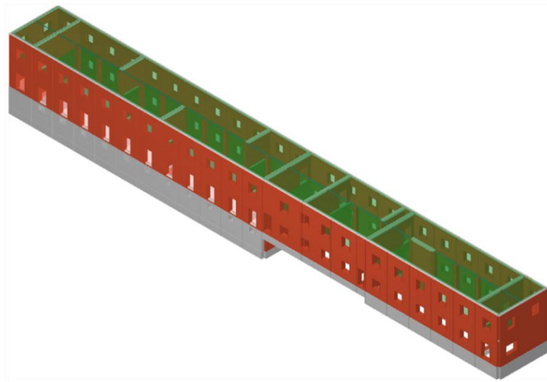
شکل ۵: مدل سه بُعدی ساختمان - تهیه شده در نرم‌افزار 3Muri Fig. 5: 3D Model of building in 3Muri software
