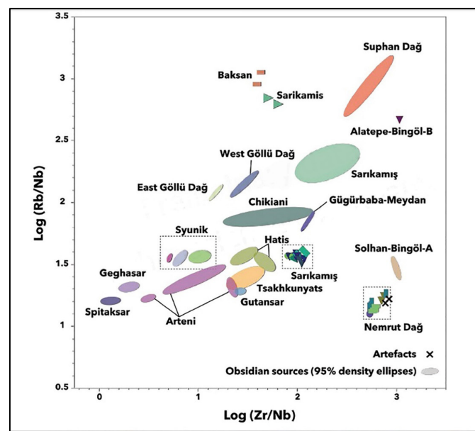
شکل ۵. نمودار مقایسه زیرکونیوم به روییدیم (Zr/Nb) و روییدیم به نیوبوم (Rb/Nb) نمونه‌های آزمایش شده تل ابلیس با دستگاه pXRF و نمونه‌های زمین‌شناسی منتخب. (با سپاس از دکتر ماریا اورنج برای تهیه نمودار فوق) Figure 5. Comparison of the (Zr/Nb) and (Rb/Nb) logratios obtained by portable XRF on the artefacts and the selected geological samples. Geological Sources: 95% density ellipses (courtesy of Dr. Maria Orange)
