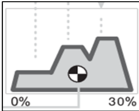
شکل ۴. نمودار خروجی سامانه حاصل از ترکیب نتیجه همه قواعد Mamdani and Sugeno Fuzzy Inference (Systems, 2024)
