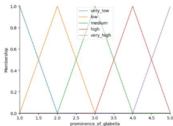
شکل ۲۲. نمودار تابع عضویت برجستگی مابین دو ابرو (Prominence of Glabella)
