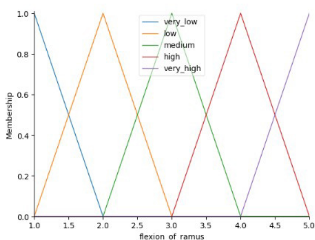
شکل ۲۱. نمودار تابع عضویت زاویه استخوان فک (Flexion of Ramus)
