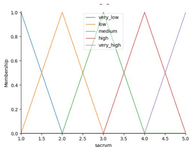
شکل ۲۰. نمودار تابع عضویت استخوان خاجی (Sacrum)
