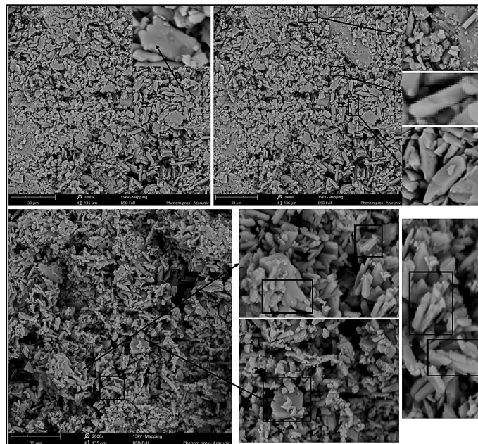
شکل ۴. مطالعه بر روی بلورهای گچی کتیبه مورد مطالعه به کمک میکروسکوپ الکترونی روبشی
