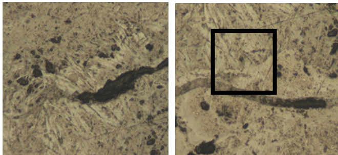
شکل ۲۳. ساختار سوزنی
