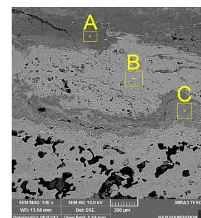
شکل ۱۹. آنالیز نقطه‌ای نمونه ۱
