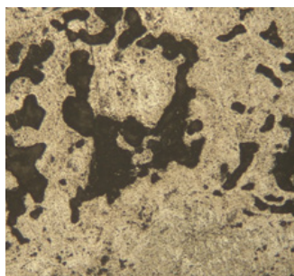
شکل ۲۲. وجود آخال‌ها
