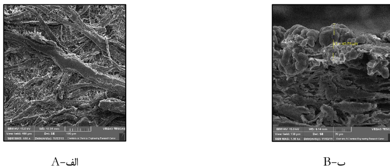
الف- A ب- B شکل ۸. آهار نشاسته: الف) کاغذ نسخه D-۳۴۵؛ ب) کاغذ نسخه T-۵۹۲۲ Figure 8. Starch sizing: A) D-345 paper and B) T-5922 paper
