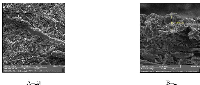
الف-الف B-ب شکل ۸. آهار نشاسته: الف) کاغذ نسخه D-۳۴۵؛ ب) کاغذ نسخه T-۵۹۲۲ Figure 8. Starch sizing: A) D-345 paper and B) T-5922 paper
