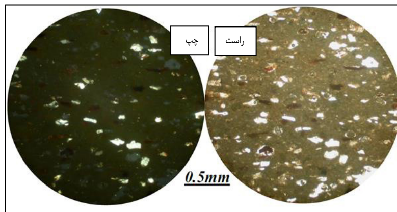
شکل ۱۱. (چپ): تصویر میکروسکوپی نمونه ۱۸، نور XPL، میدان دید 2.7 mm، بافت سیلتی، خمیره سفال در نور متقاطع کاملاً تیره و کانی کوارتز به رنگ روشن مشخص است. (راست): تصویر میکروسکوپی نمونه ۱۸، نور XPL، میدان دید 2.7 mm، بافت سیلتی، همان تصویر در نور پلاریزه است.
