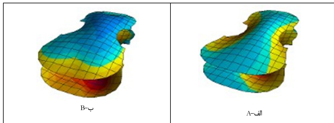
شکل ۱۱. تجزیه و تحلیل مودال ارتعاش‌های طبیعی در فرکانس‌های مشخص در بدنه‌ی ویلن ویلن ساخته‌شده توسط گوارنری. الف) ارتعاش قوی برای ۵۰۹ HZ هرتر، مد ایجاد شده توسط نت سی (B1)، ب) ارتعاش مبنای هلمهولتز برای ۲۶۸ HZ، مد ایجاد شده توسط نت لا (A0). عکس از کتاب ویوچیتا بوچور، به نقل از سایت سازندگان ویلن، Andrew Finnigam and Pia Klaembt (Bucur, 2016, p. 330)
