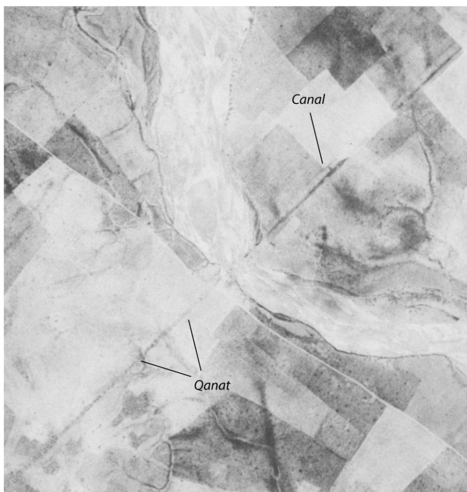
شکل ۲: بقایای سیستم آبرسانی موجود در کلار بر روی رودخانه سیروان (ماهواره کرونا)
