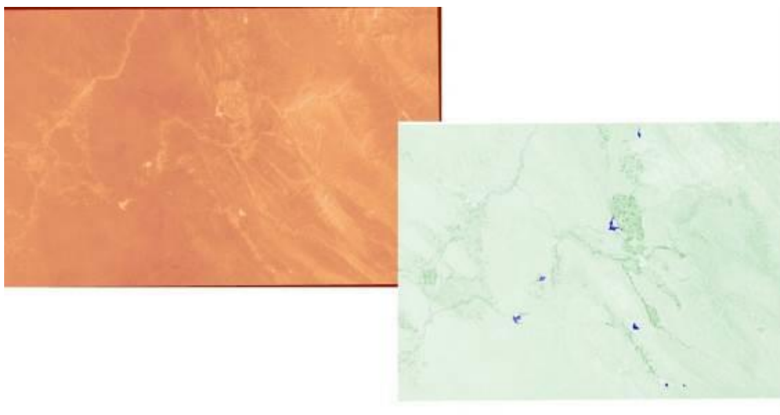
شکل ۵: راست، شاخص NDWI و چپ، شاخص Thermal در کرمانشاه و کالار (ماهواره لندست)
