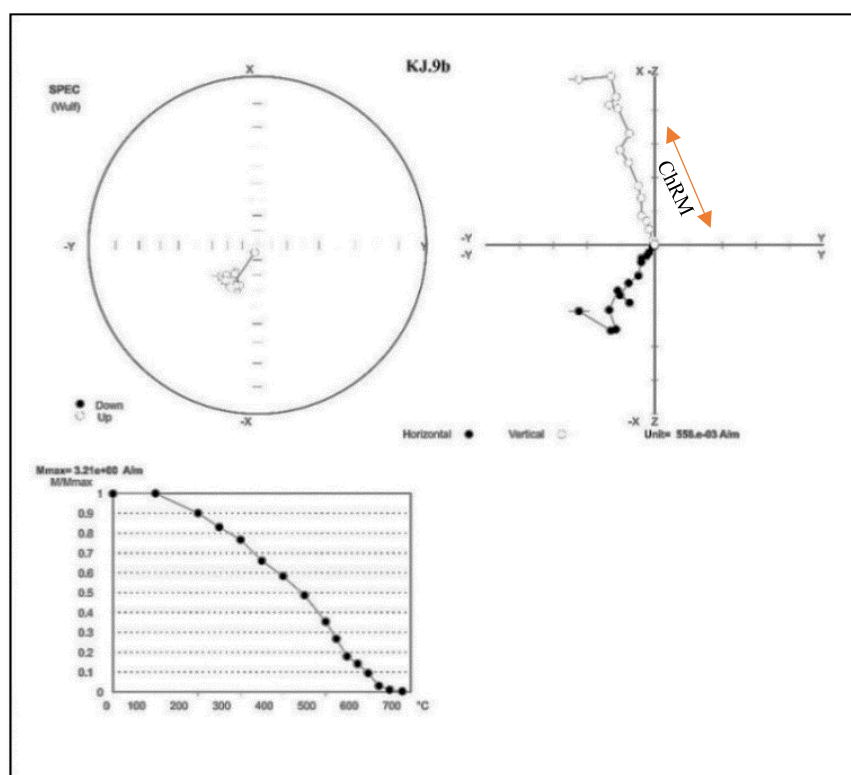
شکل ۱۰. نمودار زیجروالد نمونه K.J9 Figure 10. Zijderveld diagram of sample K.J9
