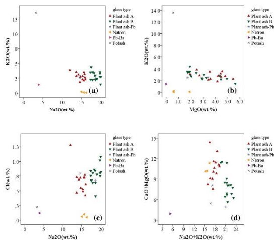
شکل ۳: a- تغییرات درصد وزنی اکسید سدیم بر حسب اکسید پتاسیم، b- تغییرات درصد وزنی اکسید منیزیم بر حسب اکسید پتاسیم، c- تغییرات درصد وزنی اکسید سدیم بر حسب کلر d- تغییرات درصد وزنی مجموع اکسید سدیم و پتاسیم بر حسب مجموع اکسید منیزیم و کلسیم در نمونه‌های آنالیز شده از تخت سلیمان و اردبیل.
