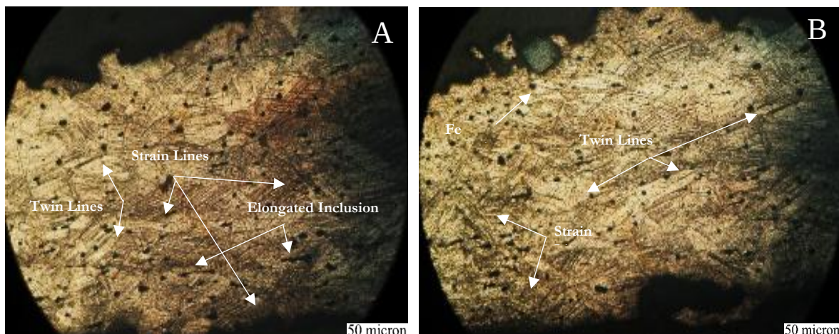
شکل ۸: ریز ساختارهای تبر (1-M) و (2-A) بعد از حکاکی در محلول \text{FeCl}_3 الکلی. در تبر شمار (1-M) شکل A و سرتبر شماره (2-A) در شکل B دانه‌های برنز متبلور و کار شده با دوقلویی و خطوط کرنش.
