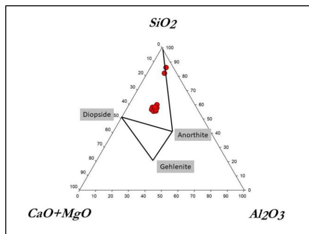
شکل ۸: نمودار طبقه‌بندی بدنه کاشی‌ها در دیاگرام نول در سیستم SiO_2 - Al_2O_3 - CaO+MgO بر اساس اندازه‌گیری
