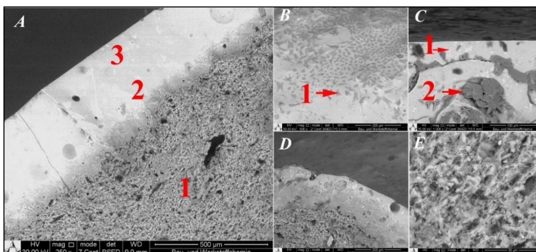
شکل ۶: A: ساختار لایه لعاب و بدنه کاشی‌ها، B: ذرات ریز منیزیم دیوپسید، C: بافت شیشه‌ای لعاب به همراه میکروکریستالیت‌های درون آن، D: بافت شیشه‌ای شده خمیر، E: حباب‌های موجود در لایه لعاب.
