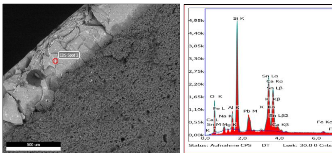
شکل ۷: طیف به دست از لعاب آنالیز شده دریکی از نمونه‌ها که وجود میزان زیاد قلع، سرب و کلسیم را نشان می‌دهد. در این لعاب، قلع به‌عنوان کورکننده، سرب به‌عنوان گدازآور و کاهش‌دهنده دمای ذوب لعاب و کلسیم به‌عنوان شبکه‌ساز استفاده شده است.
