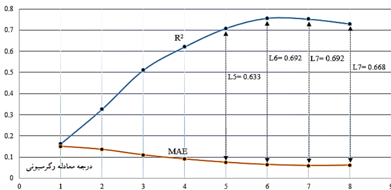
نمودار ۲: مقایسه مقادیر R2 و MAE برای هر کدام از معادلات رگرسیونی و محاسبه اختلاف میان آن‌ها Chart 2: Comparison of R2 and MAE values and calculation of the difference between regression equations
